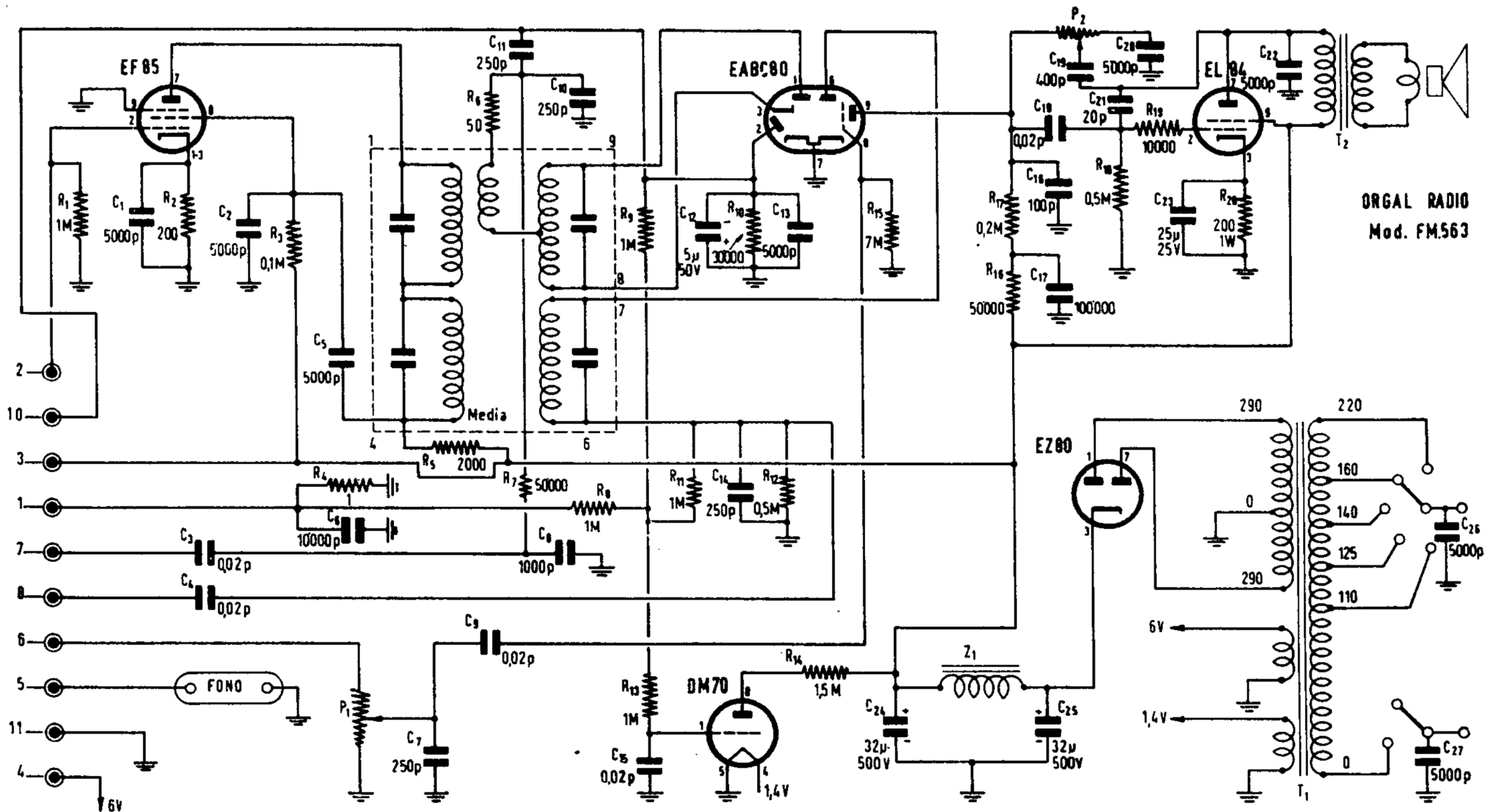
SCHEMA ELETTRICO DEL RADIORICEVITORE AM - FM, ORGAL, MOD. FM563
